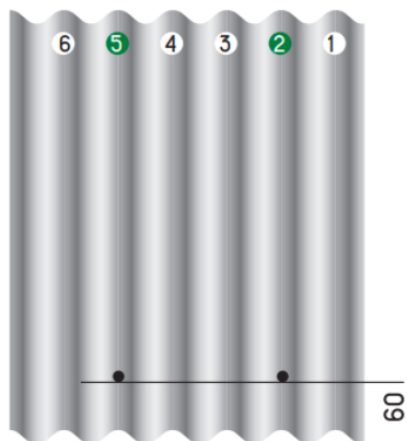
Установка крепежного элемента на лист СЕ
