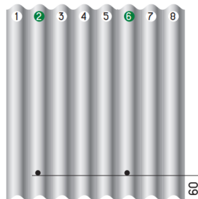
Установка крепежного элемента на лист СВ
