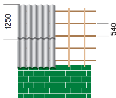
Рекомендуемое расположение листа СЕ на обрешетке
