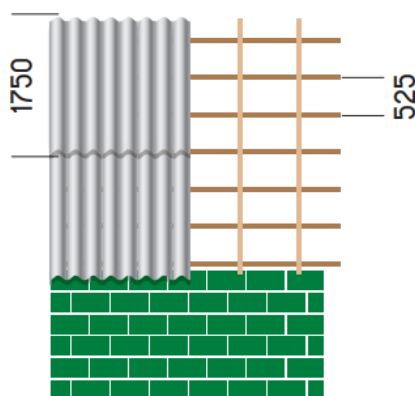
Рекомендуемое расположение листа СВ на обрешетке
