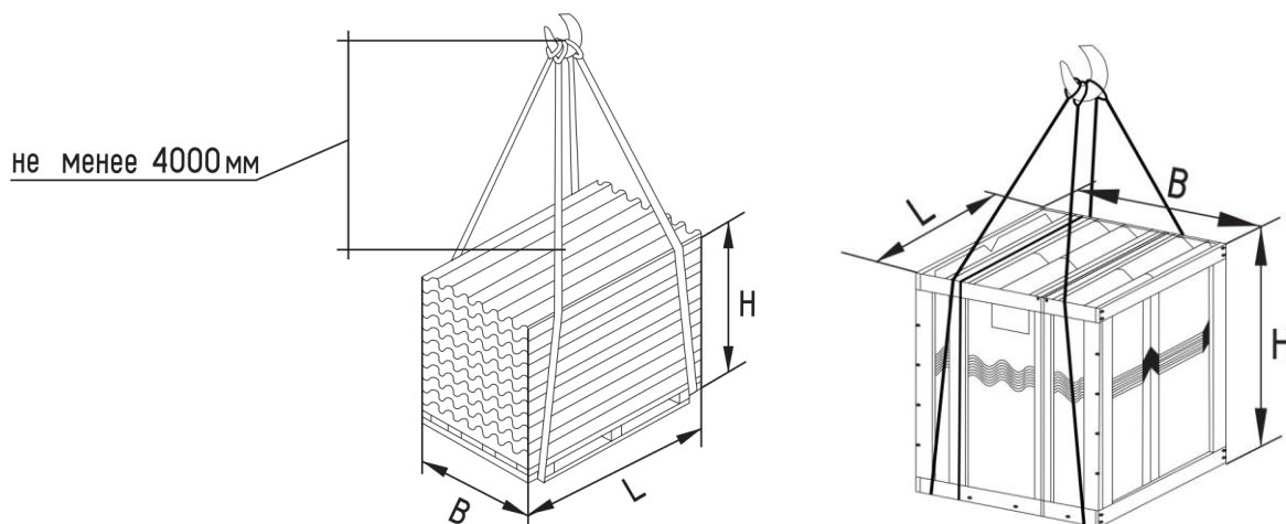
Строповка пакета стропами (В-ширина пакета, L-длина пакета, Н – высота пакета)
