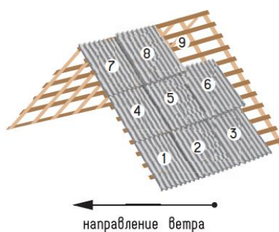
Укладка листов слева направо
