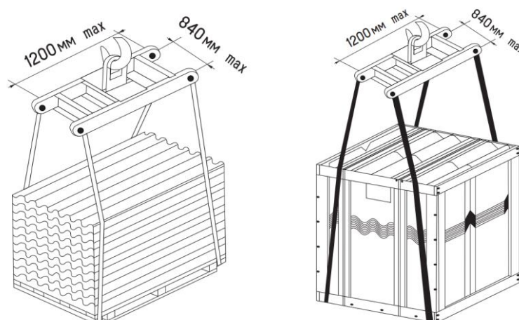
Строповка пакета траверсой со стропами
