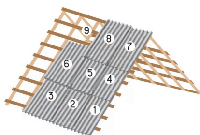
Схема укладки листов СЕ
