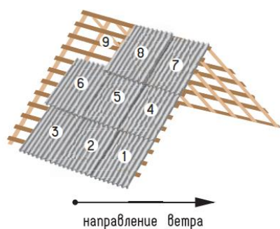
Схема укладки листов СВ
