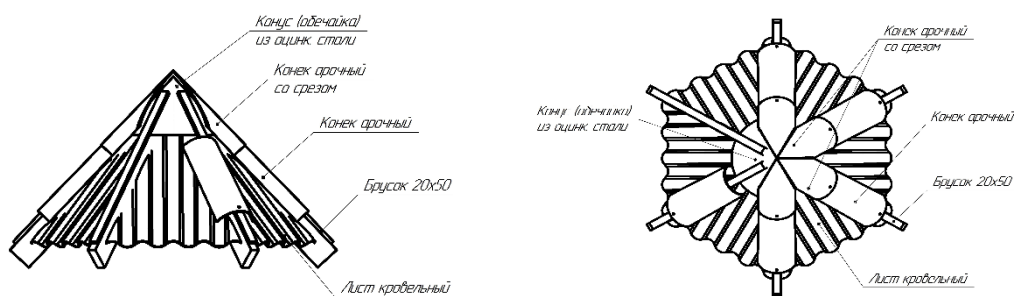
Крепления детали арочной коньковой для шатровой крыши
